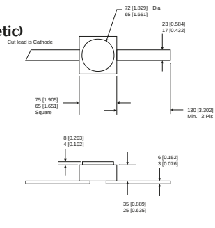
H40 (hermetic)
